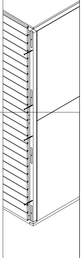
Abbildung 2.2b. Eckbefestigung
